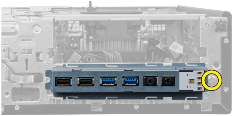
7. أخرج لوحة الإدخال/الإخراج باتجاه الجانب الأيسر من الكمبيوتر لتحريره، واسحب للوحة الإدخال/الإخراج (I/O) مع الكبل الخاص بها إلى خارج الكمبيوتر.
